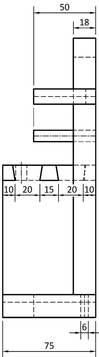
End View/Taobhchló
