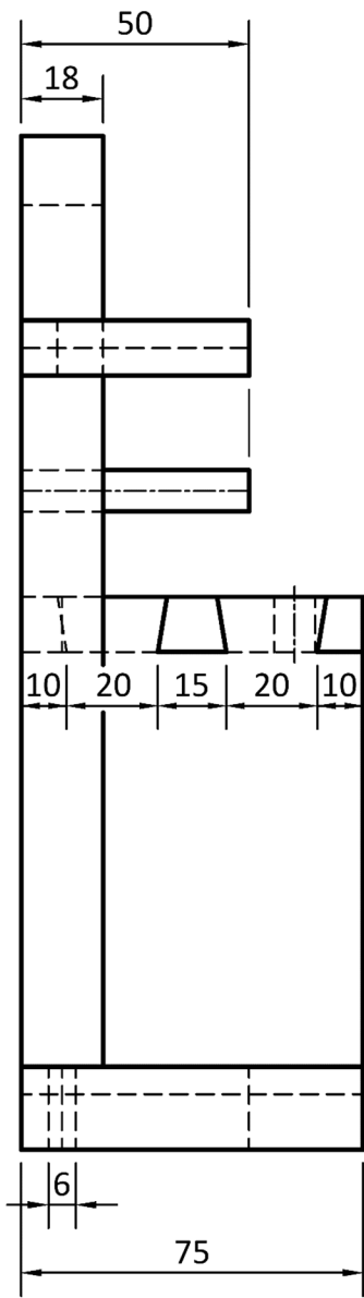
End View/Taobhchló
