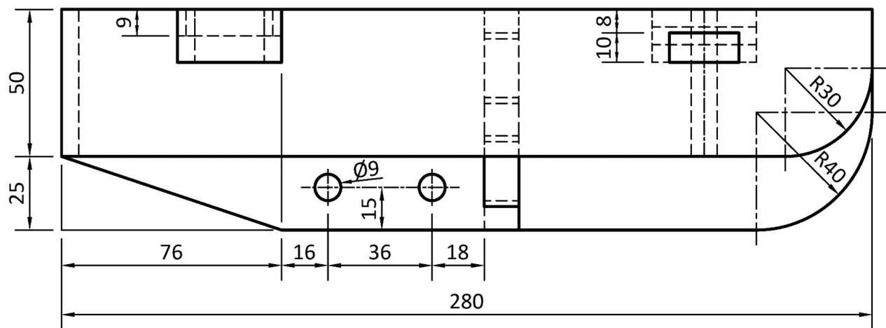
Plan/Bonnchló
